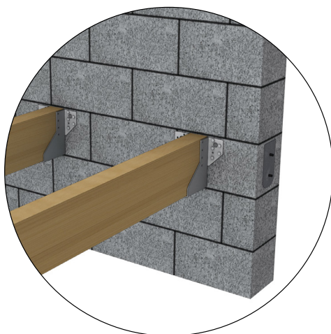
Sabot métallique
