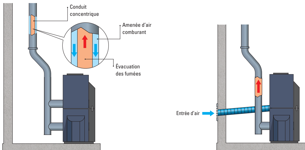
FIGURE 1 Exemples de configurations possibles pour une installation à circuit de combustion étanche. À gauche par un conduit concentrique, à droite par conduits séparés.
