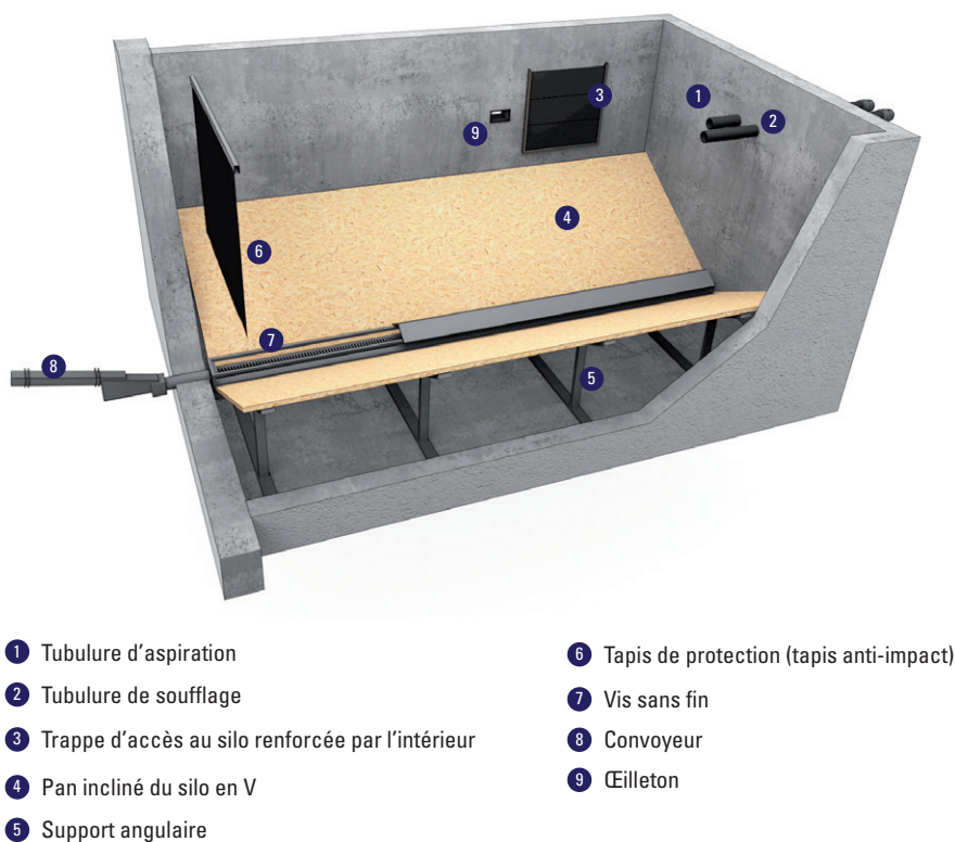
FIGURE 3 Illustration d'un silo en V avec vis sans fin d'extraction
