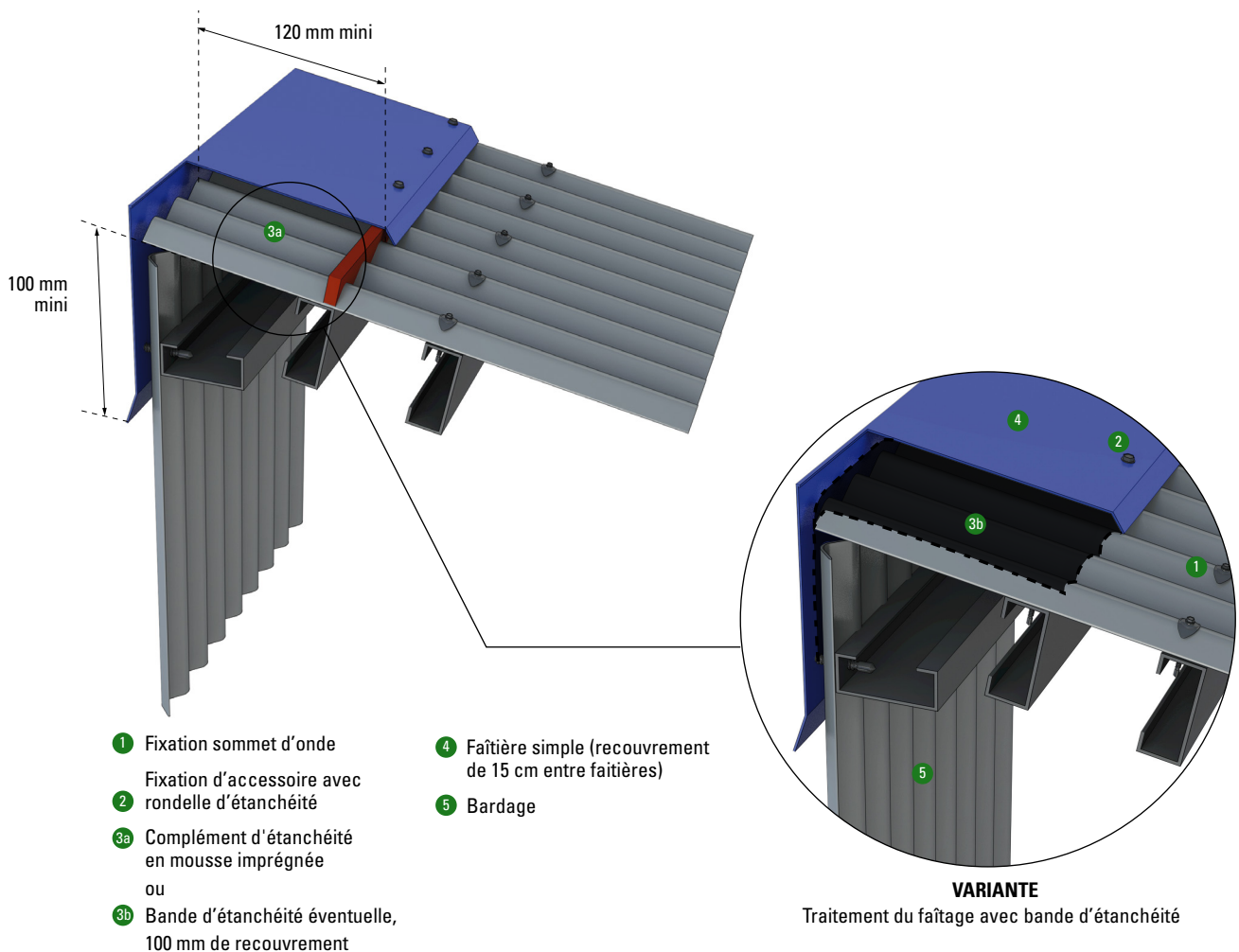
Figure 45 – Faîtage simple (monopente)
