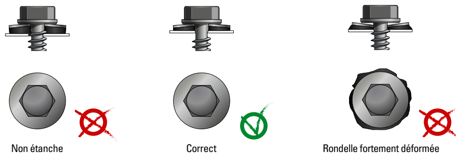
Figure 42 – Serrage des fixations des accessoires
