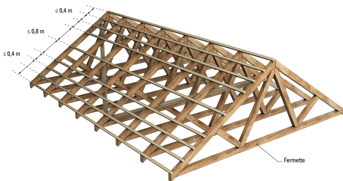
Figure D4 – Espacement des linteaux fixés à une charpente industrialisée type fermettes
