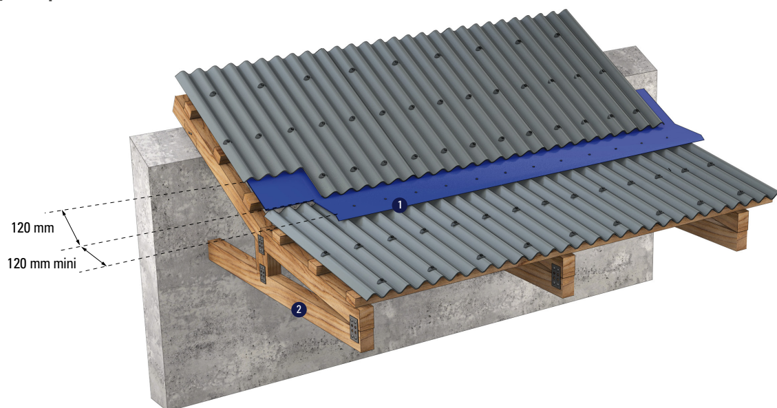
Figure 53 – Désolidarisation des ouvrages annexes hors zones cycloniques
