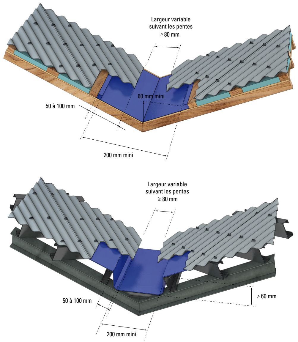
Figure 50 – Noue encaissée (coupe dans le sens de la pente)
