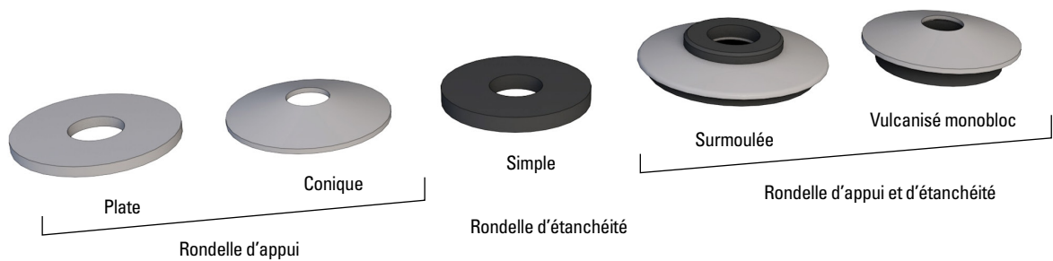
Figure 14 – Exemples d'accessoires de vis de couture
