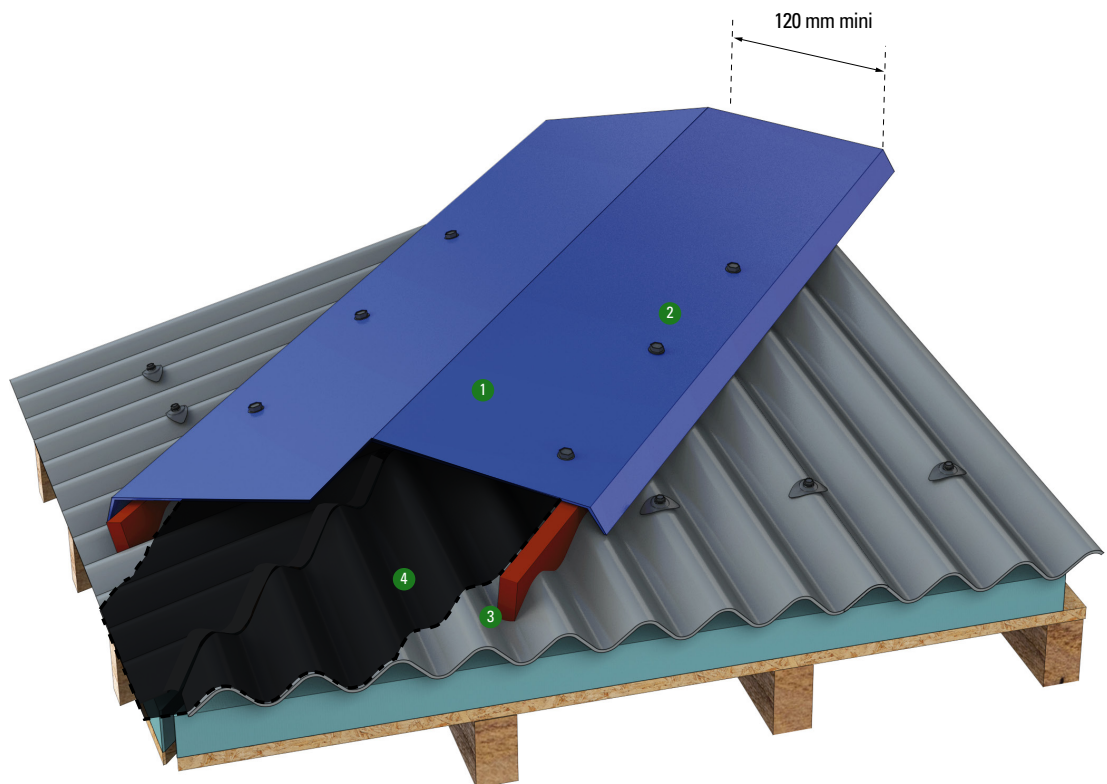
Figure 49 – Arêtier
