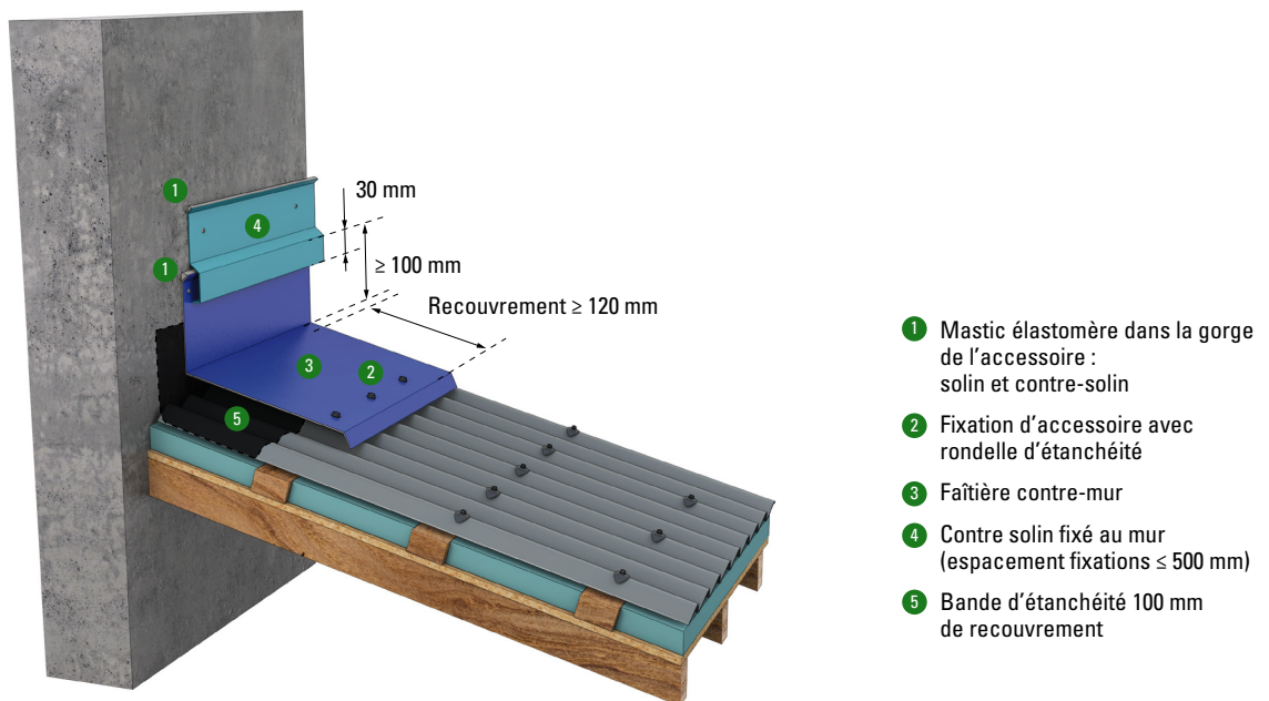
Figure 46 – Faîtage contre mur
