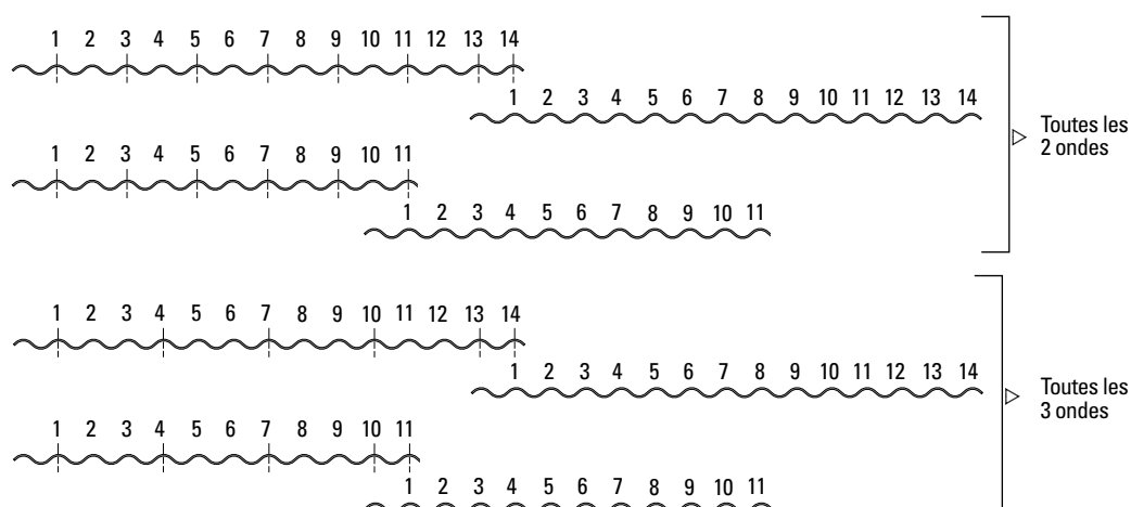
Figure 37 – Positionnement et densité des fixations aux recouvrements en zone cyclonique
