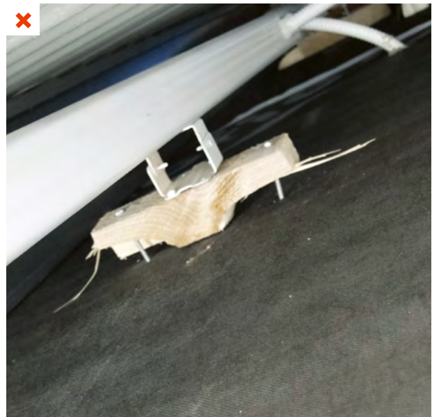
Exemple de détérioration d'une membrane d'étanchéité à l'eau par un opérateur du second œuvre : les pointes servant à fixer les cales qui supportent le réseau électrique percent le pare-pluie. ©AQC
