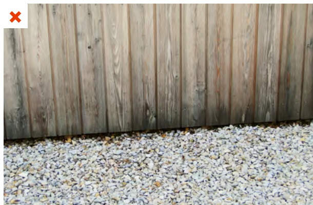
Le problème ici n'est pas normatif comme ci-dessus car le sol est drainant (gravier), cependant le bardage est tout de même trop près du sol empêchant une ventilation suffisante de la lame d'air (entraînant un noircissement). ©AQC
